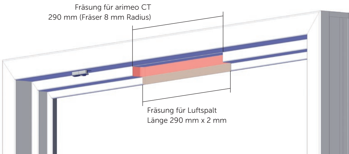
Abbildung 1: Fräsung
